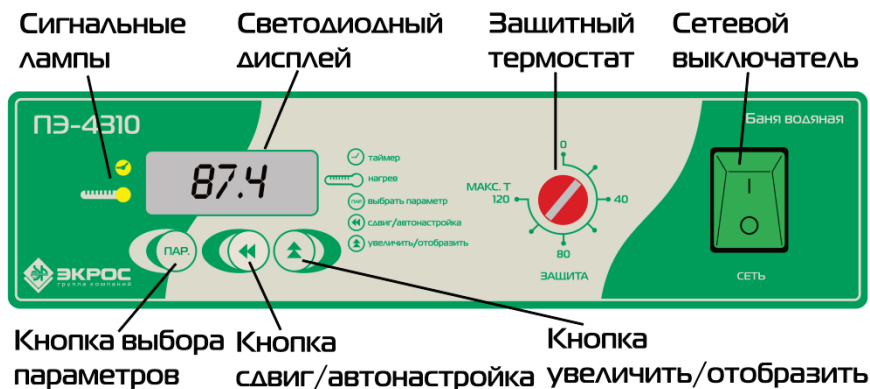
Рисунок 2 – Панель управления
